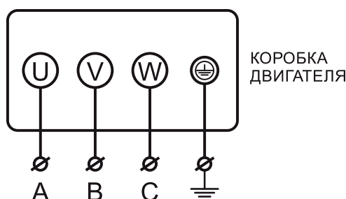
Рисунок 6.2 – Клеммная коробка двигателя
